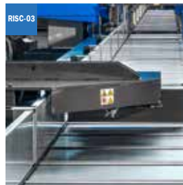
RISC-03 Riscontro motorizzato con scorrimento su profilo in acciaio e sollevamento idraulico Powered length stop with sliding on iron pipe with encoder and hydraulic lifting
